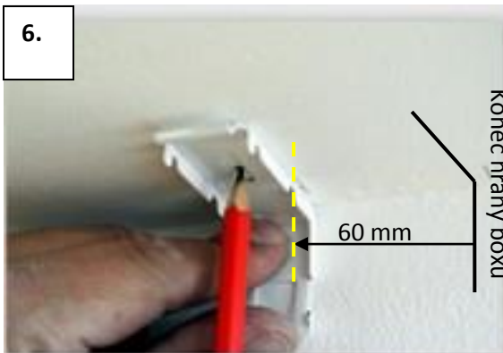
Montáž konzoly 60 mm od hrany boxu.
