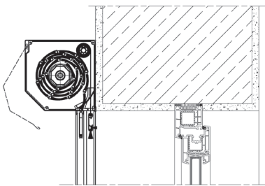
A Roleta namontovaná na stěně budovy. Roleta navíjená směrem ven (levotočivá)
