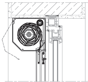
B Roleta namontovaná v okenním otvoru. Roleta navíjená směrem ven (levotočivá)
