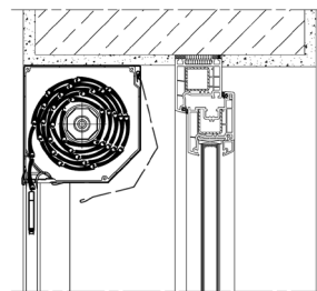
C Roleta namontovaná v okenním otvoru. Roleta navíjena směrem dovnitř (pravotočivá)
