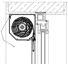
B Roleta namontovaná v okenním otvoru. Roleta navíjena směrem ven (levotočivá)
