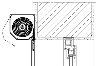
A Roleta namontovaná na stěně budovy. Roleta navíjena směrem ven (levotočivá)
