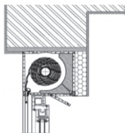
B Skříňka rolety zabudovaná zevnitř objektu, otevíraná zespodu
