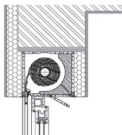
C Skříňka rolety zabudovaná z vnějšku i zevnitř objektu, otevíraná zespodu
