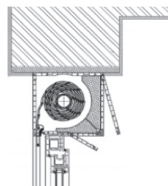
D Skříňka rolety bez zabudování, otevíraná zespodu nebo zepředu
