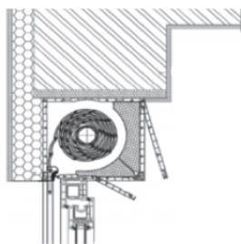
A Skříňka rolety zabudovaná z vnějšku objektu, otevíraná zespodu nebo zepředu
