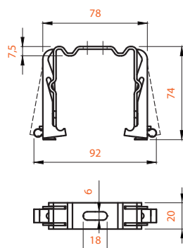
Pružinový bez gumy
