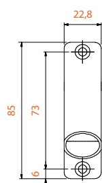
Průchodka 90°
