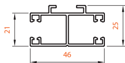
VL3 Středová 46 × 25 mm
