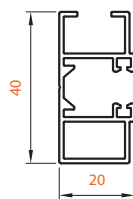
VL6 Samonosná 20 × 40 mm
