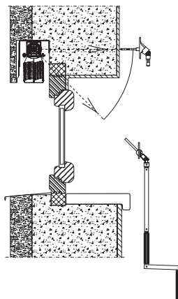
A Dodatečná montáž. Žaluzie namontovaná na stěně budovy.
